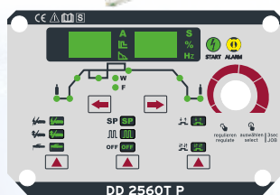
Bedienpanel DD 2560T P
